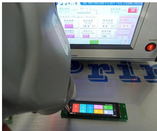
图 3-2 ESD 测试图
