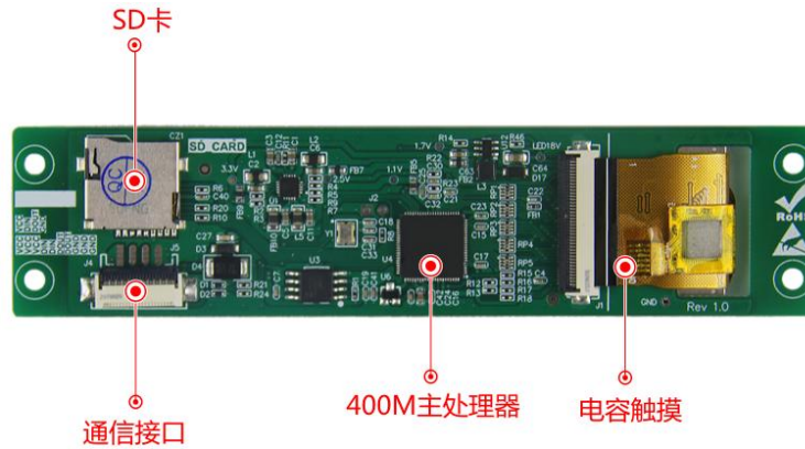
图 1-2 硬件配置图
